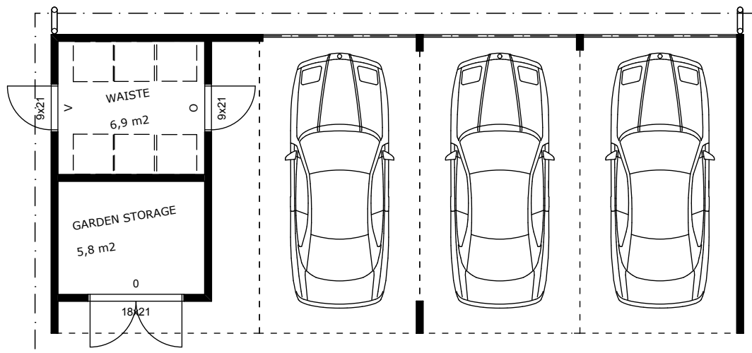
PLAN 1:100
