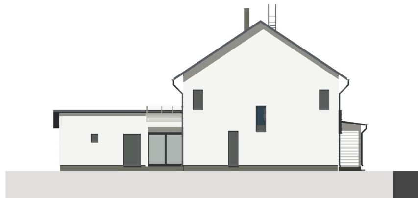
ETELÄÄN
