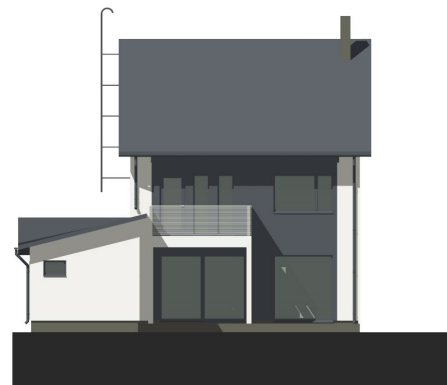
POHJOISEEN
