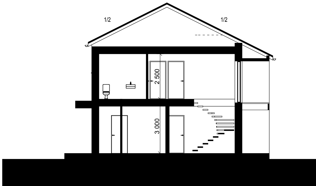
LEIKKAUS A-A
