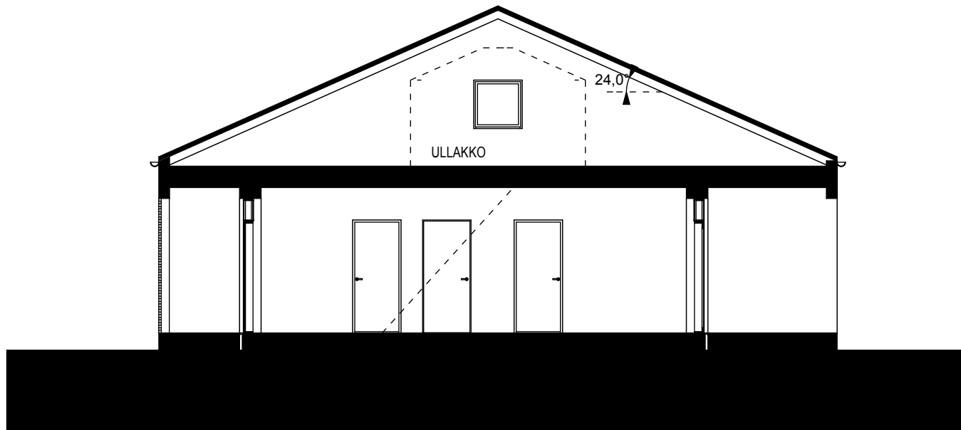
LEIKKAUS A-A
